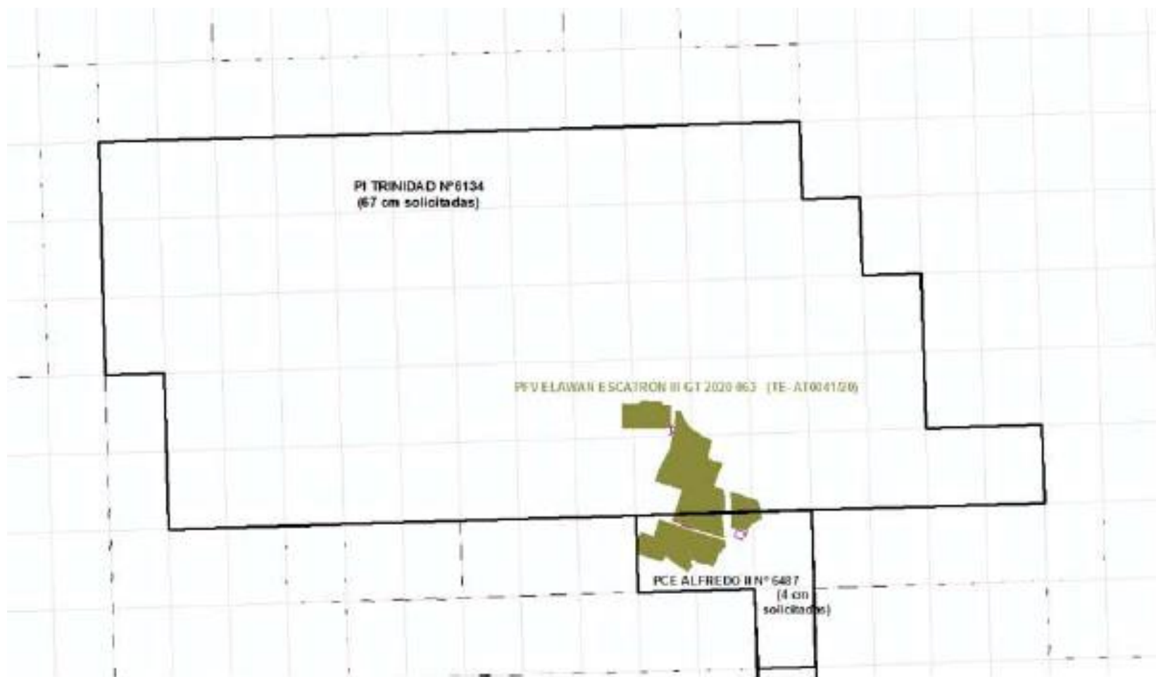
Plano n°1. Derechos Mineros que afectan a la PFV ELAWAN ESCATRÓN III G-T-2020-063 (TE-AT0041/20)
